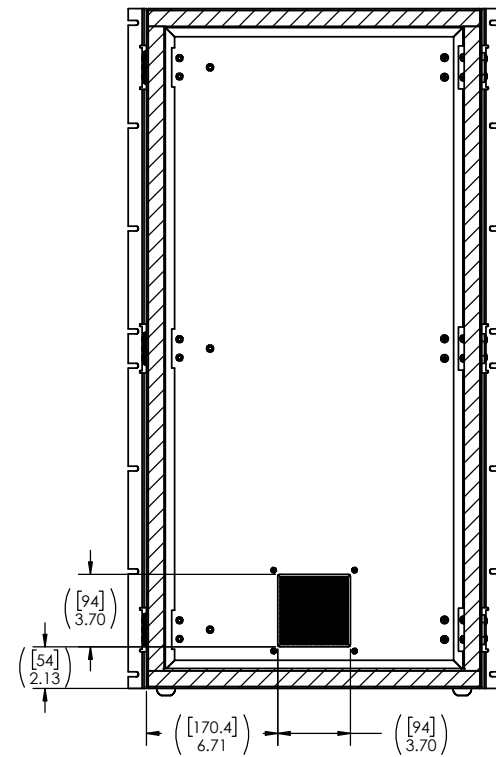
SECTION E-E SCALE 1 : 4.9
