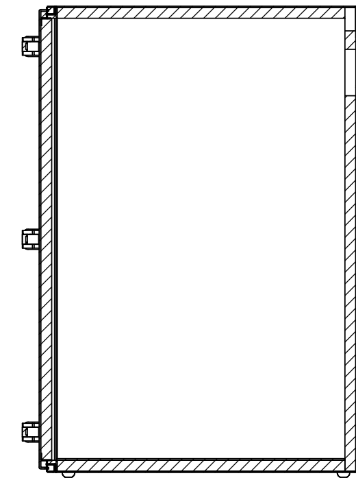
SECTION D-D SCALE 1 : 4.9
