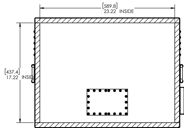
SECTION D-D
